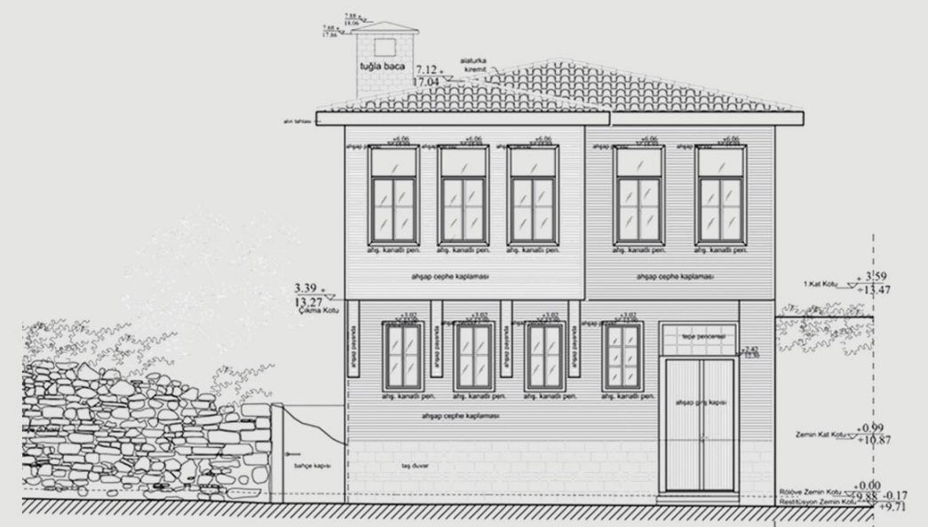
EYÜPSULTAN AHŞAP SİVİL YAPI RESTİTÜSYON ÇİZİMİ
