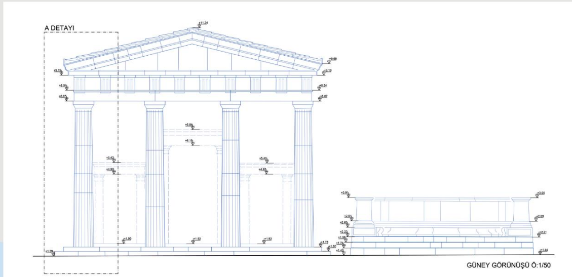
RESTİTÜSYON ÇİZİMLERİ
