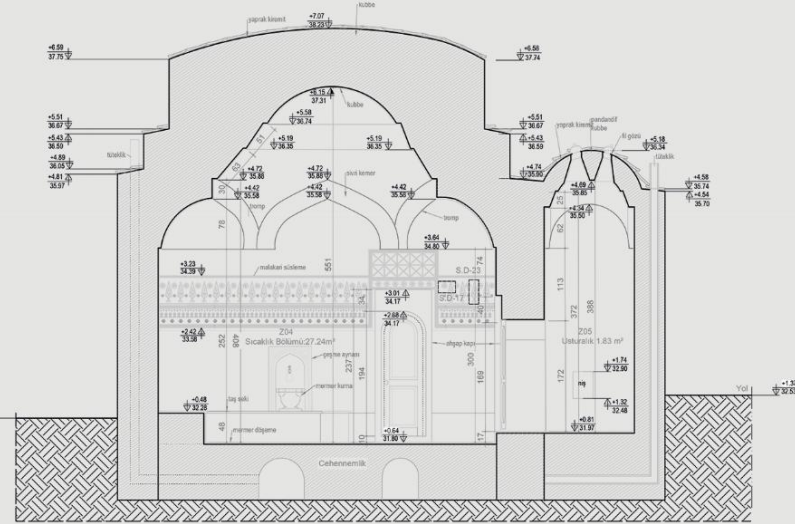
C-C KESİTİ
