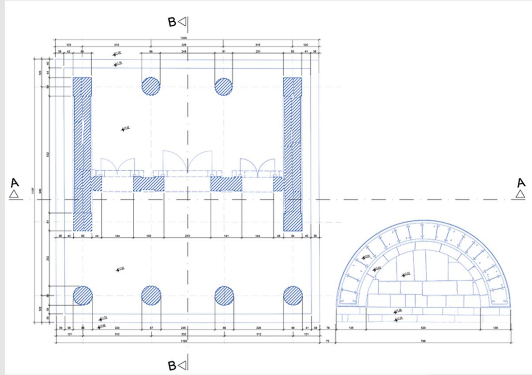
RESTİTÜSYON ÇİZİMLERİ
