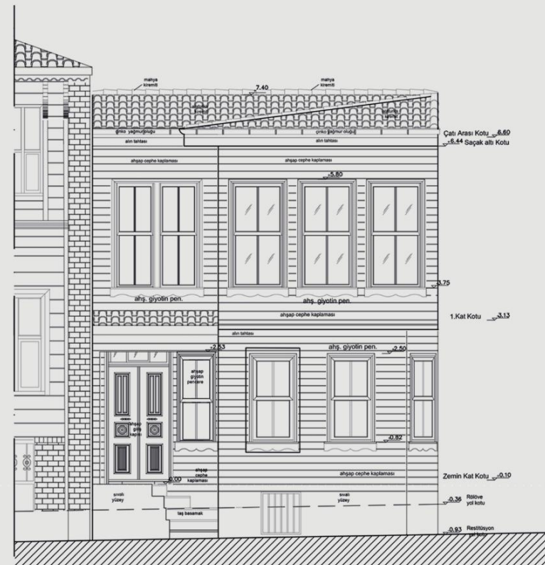
EYÜPSULTAN AHŞAP SİVİL YAPI RESTİTÜSYON ÇİZİMİ
