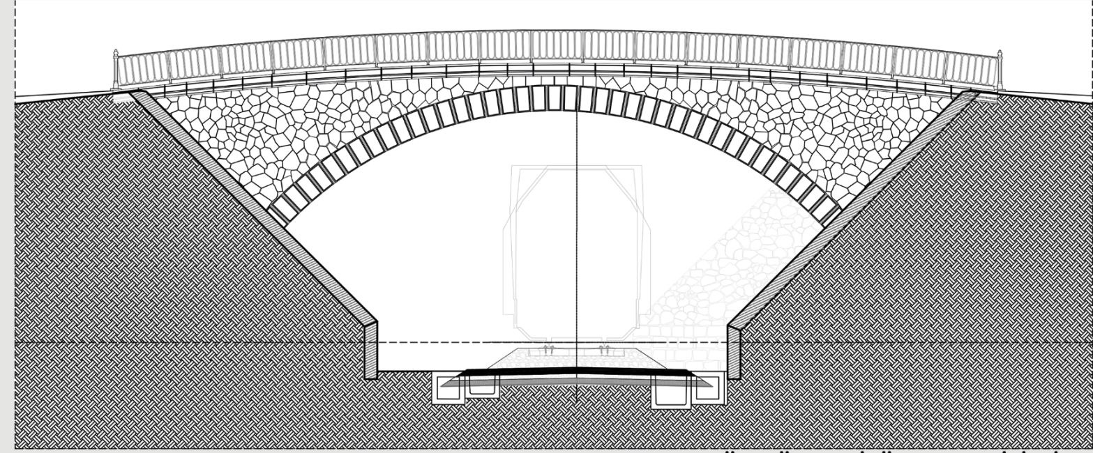
TAŞ KÖPRÜ RESTİTÜSYON ÇİZİMİ
