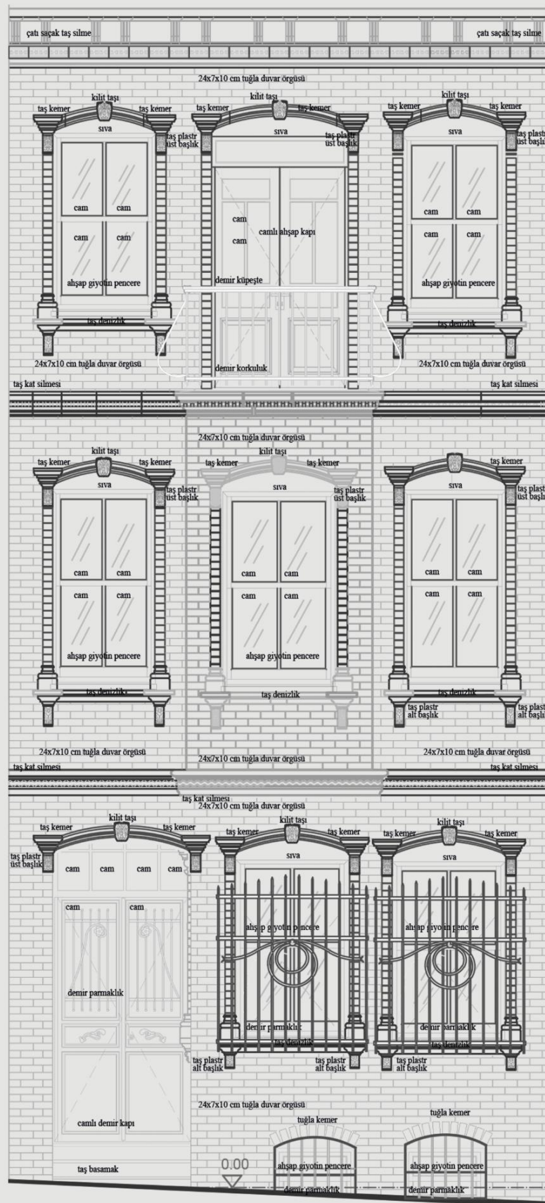
YELDEĞİRMENİ PROJESİ RESTİTÜSYON ÇİZİMİ
