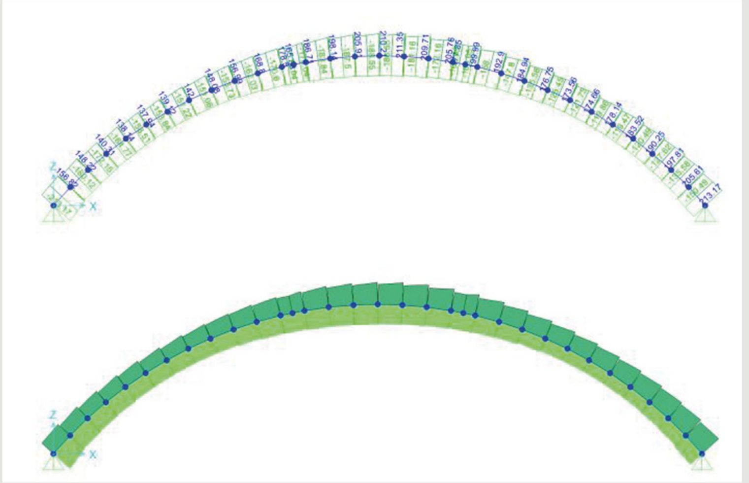
TARİHİ MENFEZYAPISI STATİK DİAGRAMI
